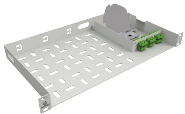
Tiroirs de rangement 1U 12 Ports SC
